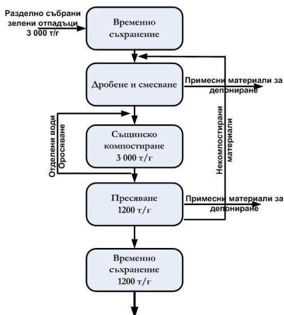
Фигура 5. Технологична блок схема на Инсталацията за компостиране ИНСТАЛАЦИЯ ЗА КОМПОСТИРАНЕ
