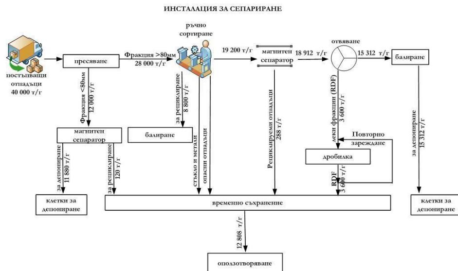
Фигура 4. Технологична блок схема на Инсталацията за сепариране
